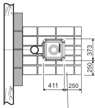
КИРПИЧНОЕ ОСНОВАНИЕ ДЛЯ УСТАНОВКИ ПЕЧИ
